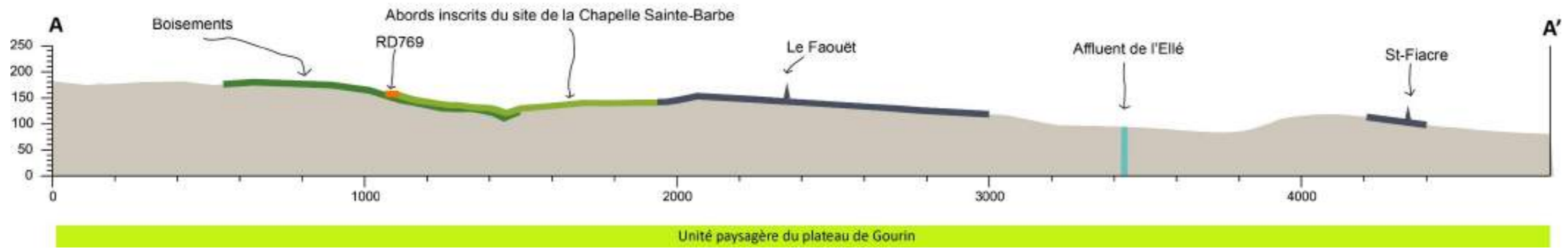
Figure 26 : La coupe topographique AA' – Augmentation altimétrique x1,7
