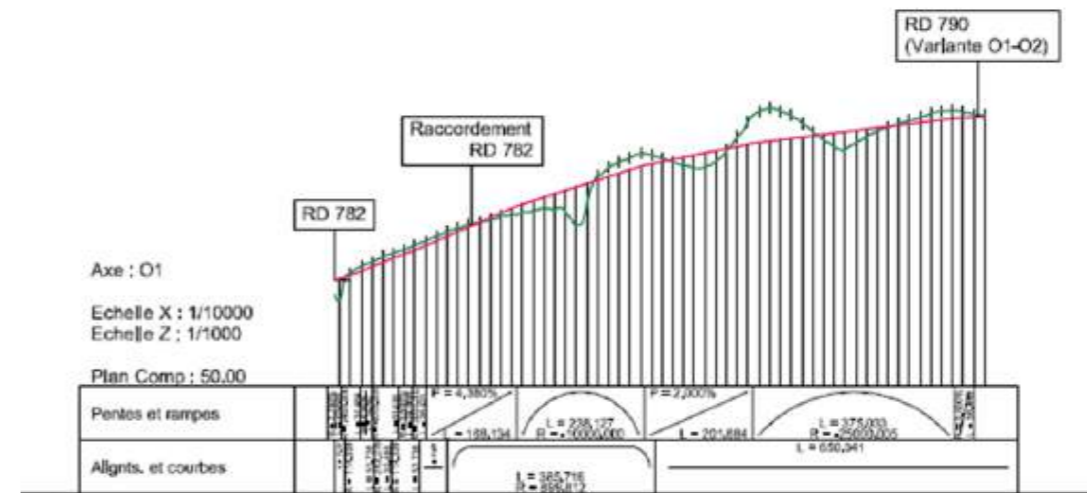
Carte 201 : Extrait de l'étude d'opportunité – profil en long de O1.
