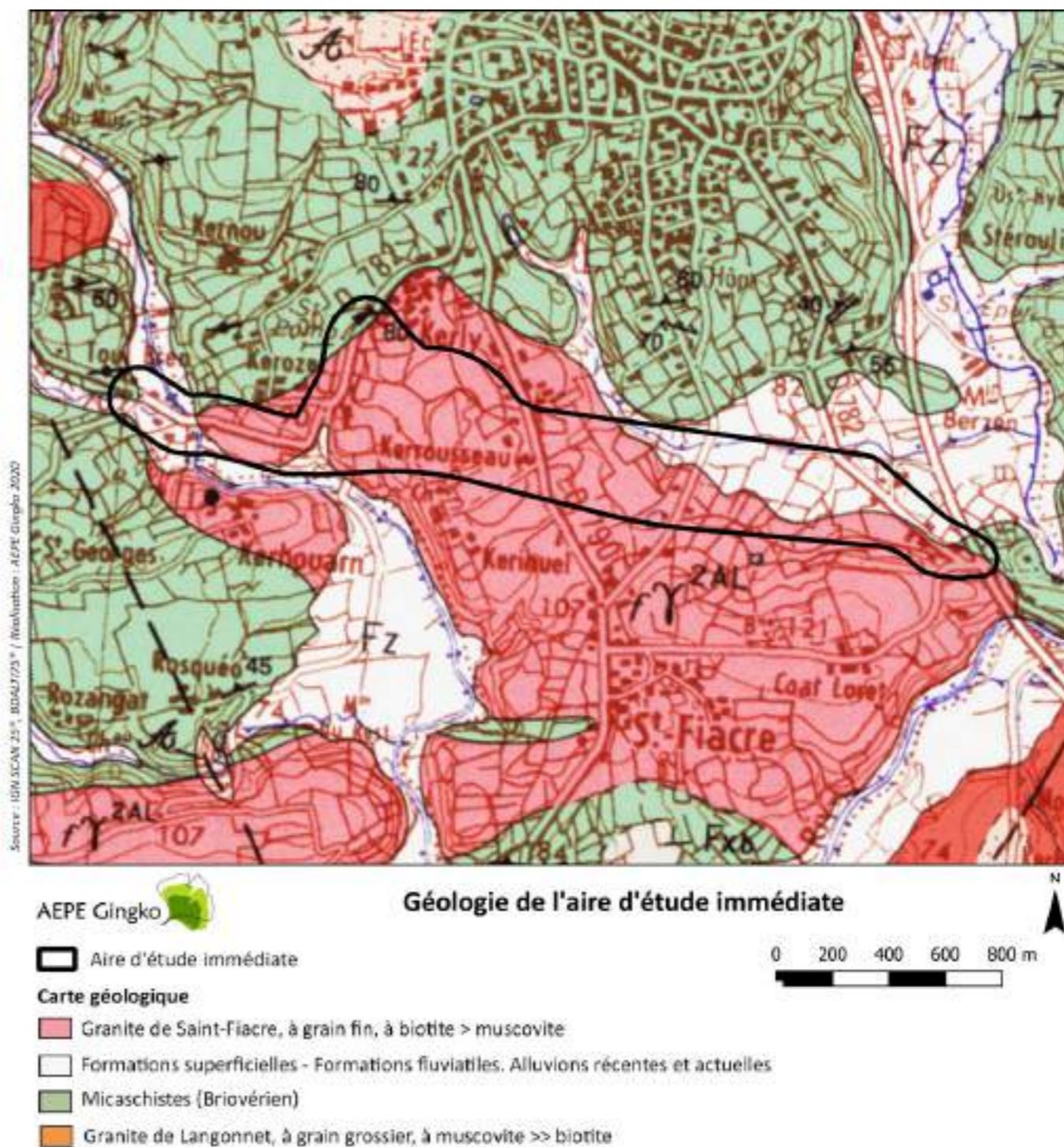
Carte 12 : Carte géologique de l'aire d'étude immédiate
