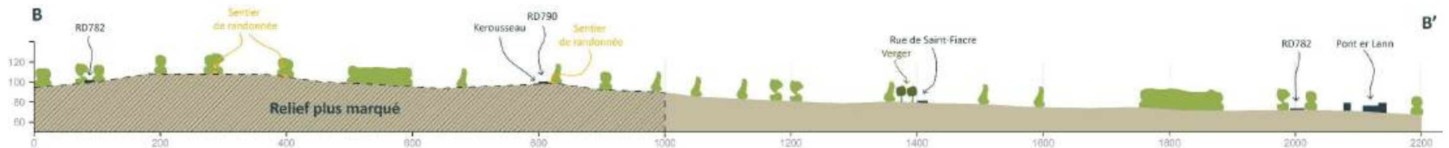
Figure 32 : Coupe BB' à l'échelle du fuseau retenu – Augmentation altimétrique x1,6
