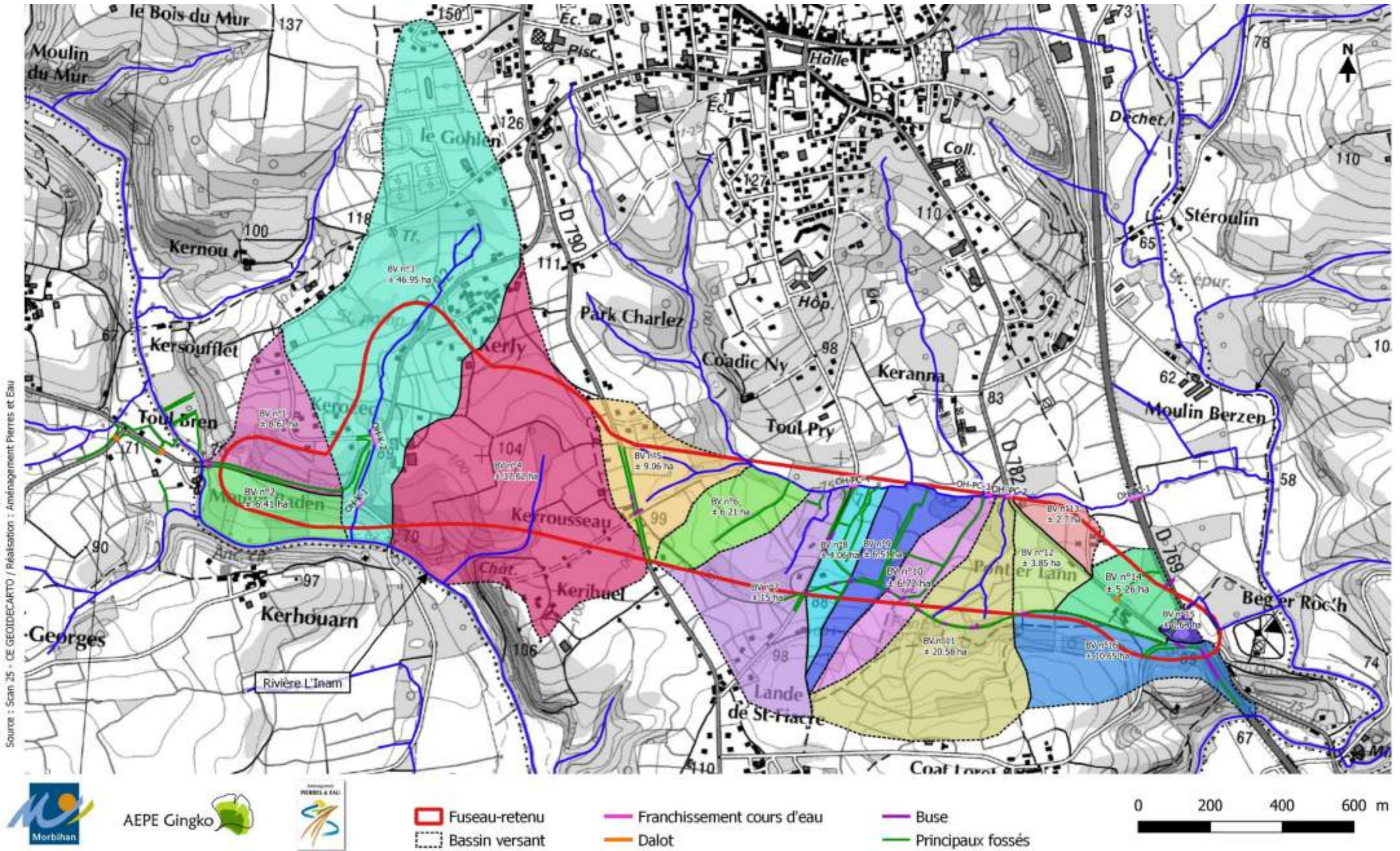
Carte 22 : Bassins versants naturels et ouvrages hydrauliques existants
